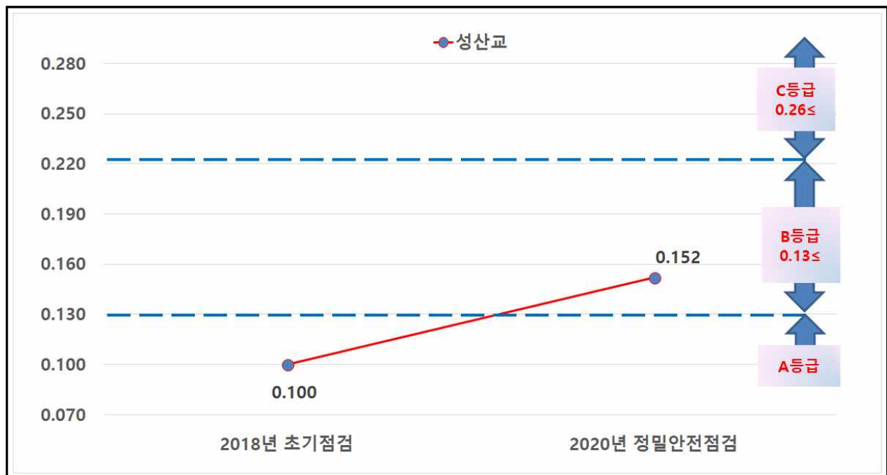
[그림 5.4.1] 성산교 상태평가 결과 비교 그래프
